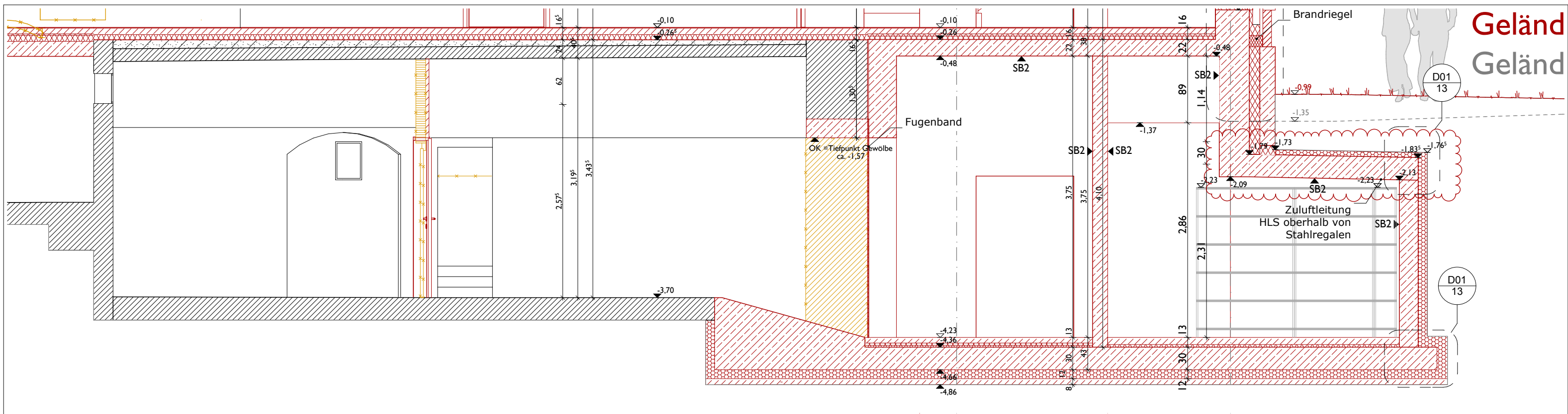
AUSSCHNITT SCHNITT L1 1:50
