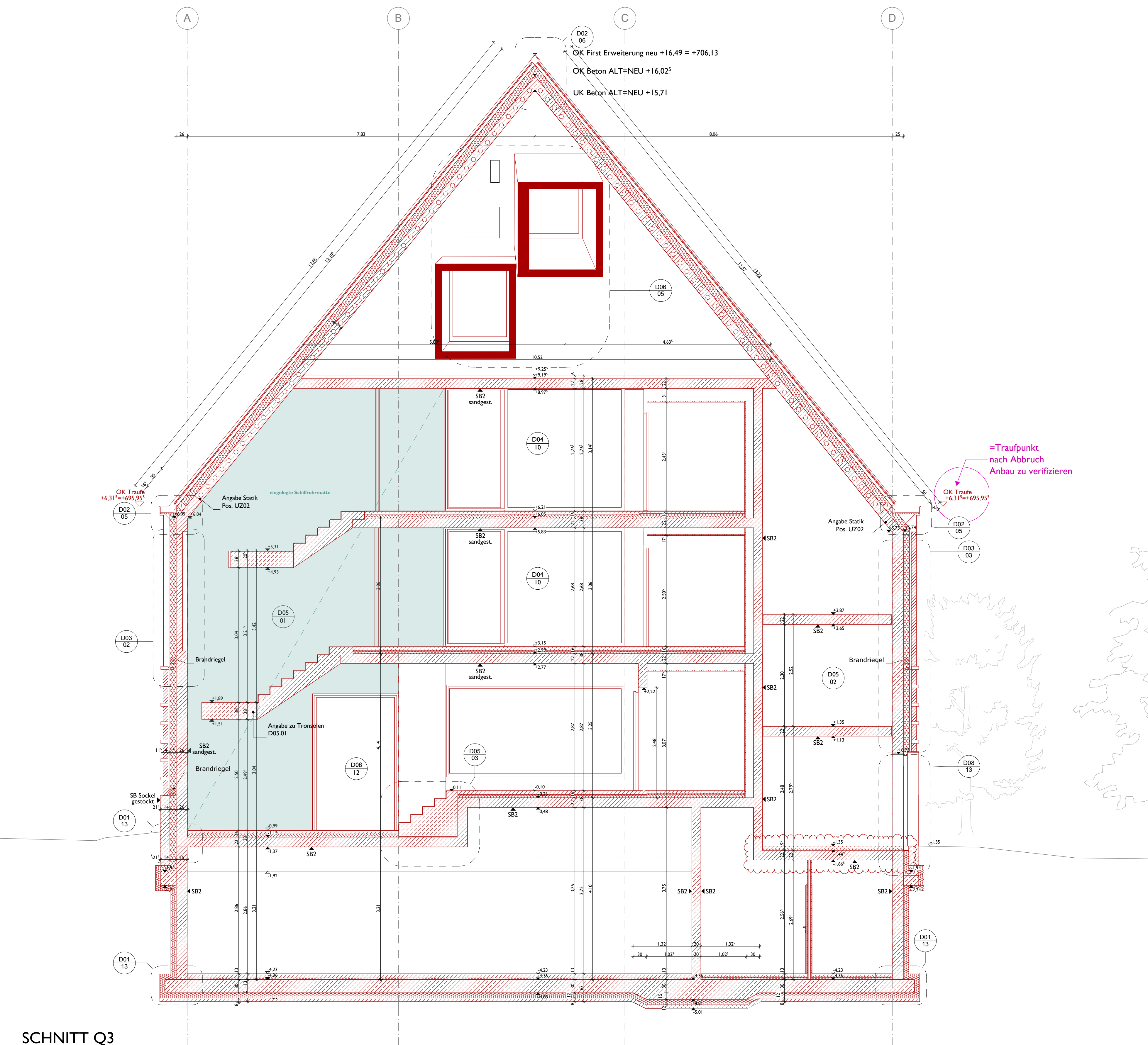
SNITT Q3
