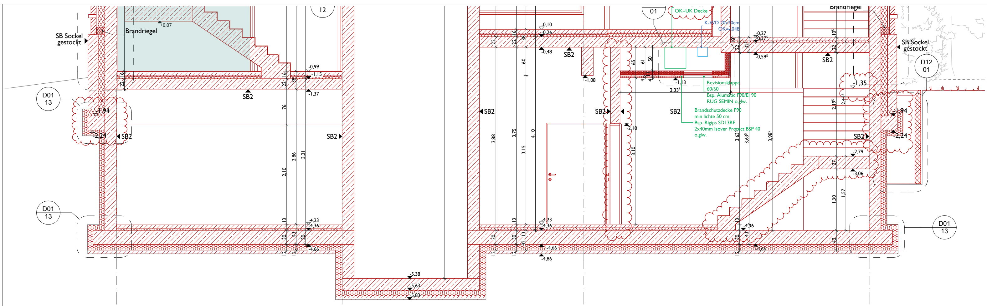
AUSSCHNITT SCHNITT Q4 1:50
