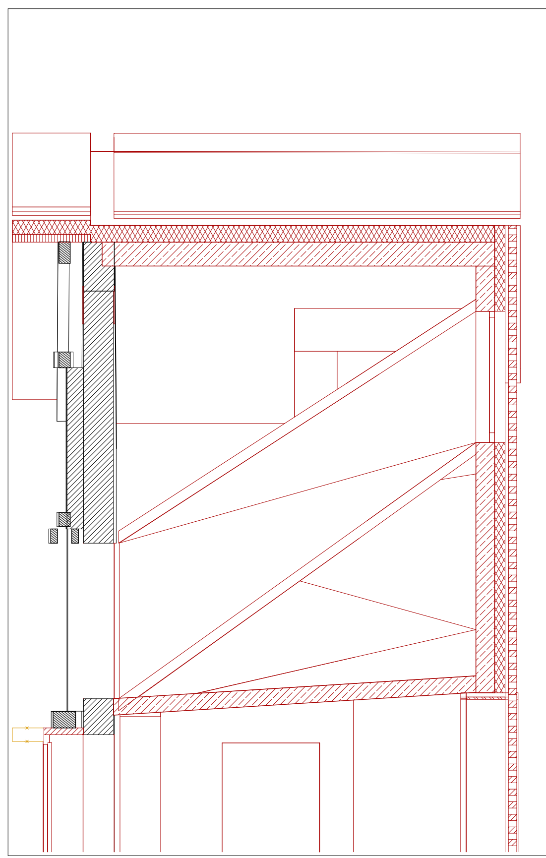
SNITT_TECHNIK 02 1:50
