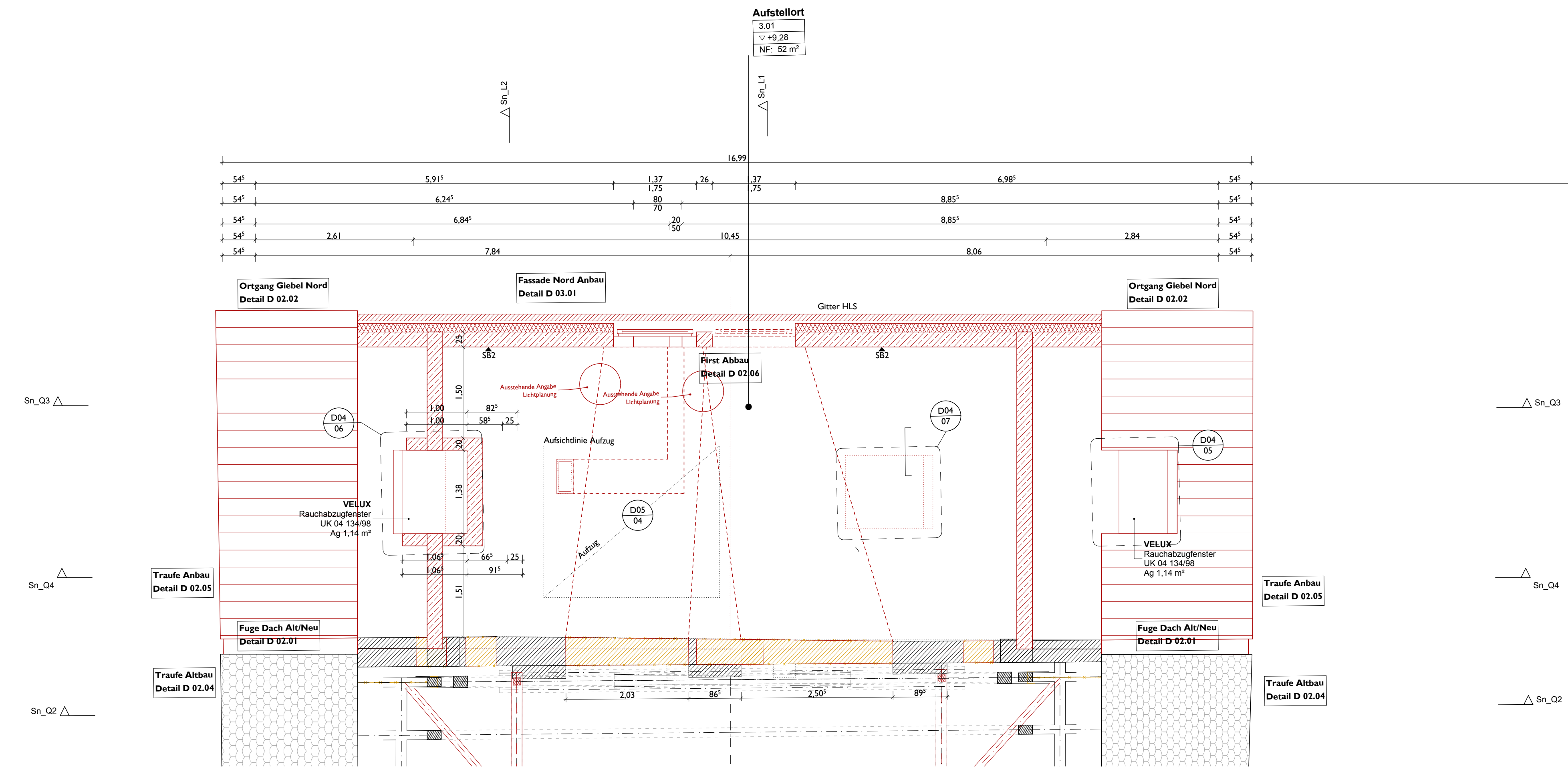
TECHNIKESCHOSS SNITT ÜBERSICHT 1:50
