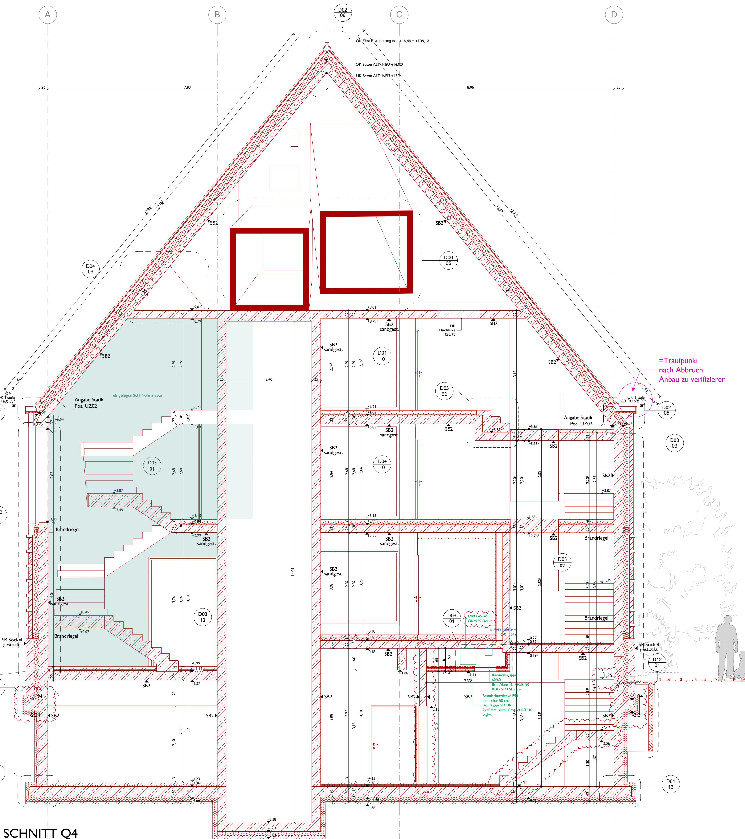
SNITT Q4
