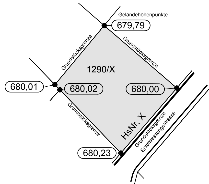
Beispiel Grundstück M 1: 500 mit Geländehöhenpunkte (Höhenangabe über Normal Null)
